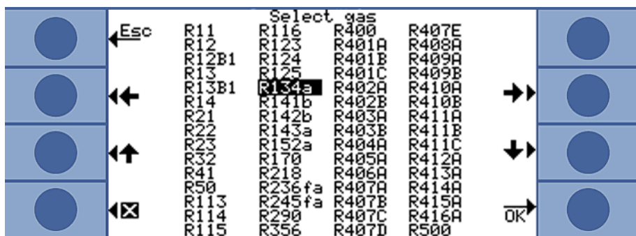
Abb. 21: Biblioteka gazów
