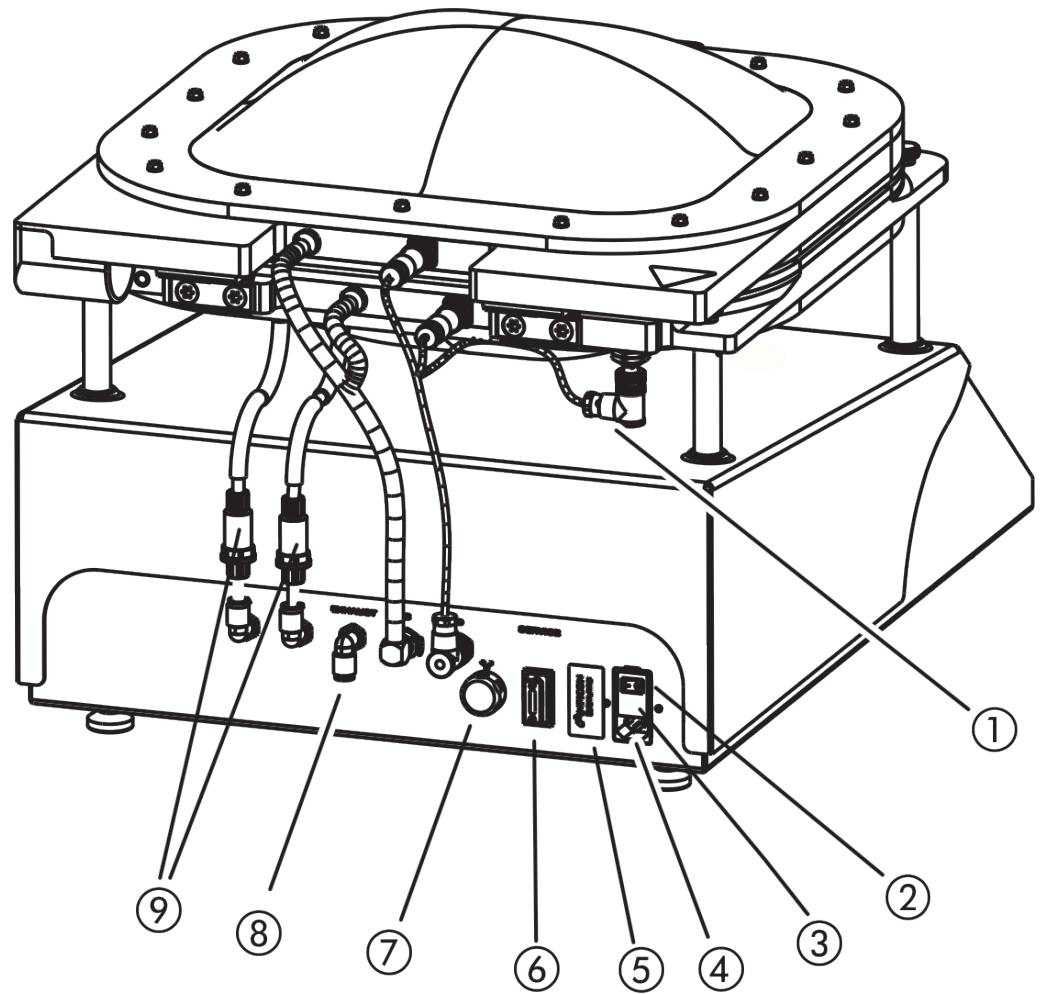
插图 2: 后视图
