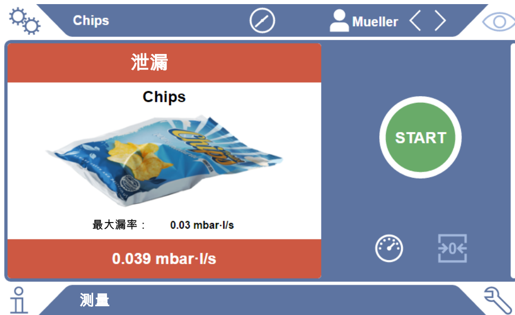
插图 4: 以红色背景显示的测量结果，对应于高漏率
